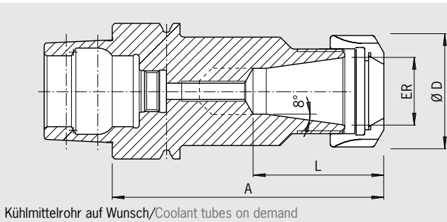
Kühlmittelrohr auf Wunsch/Coolant tubes on demand
